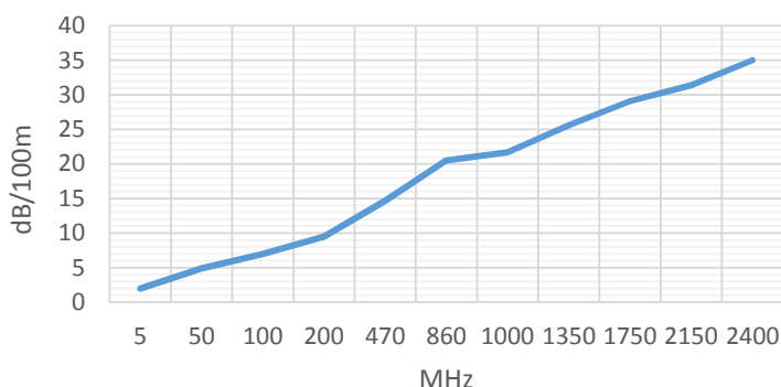
charakteristika útlumu při 20 ^{\circ} C
